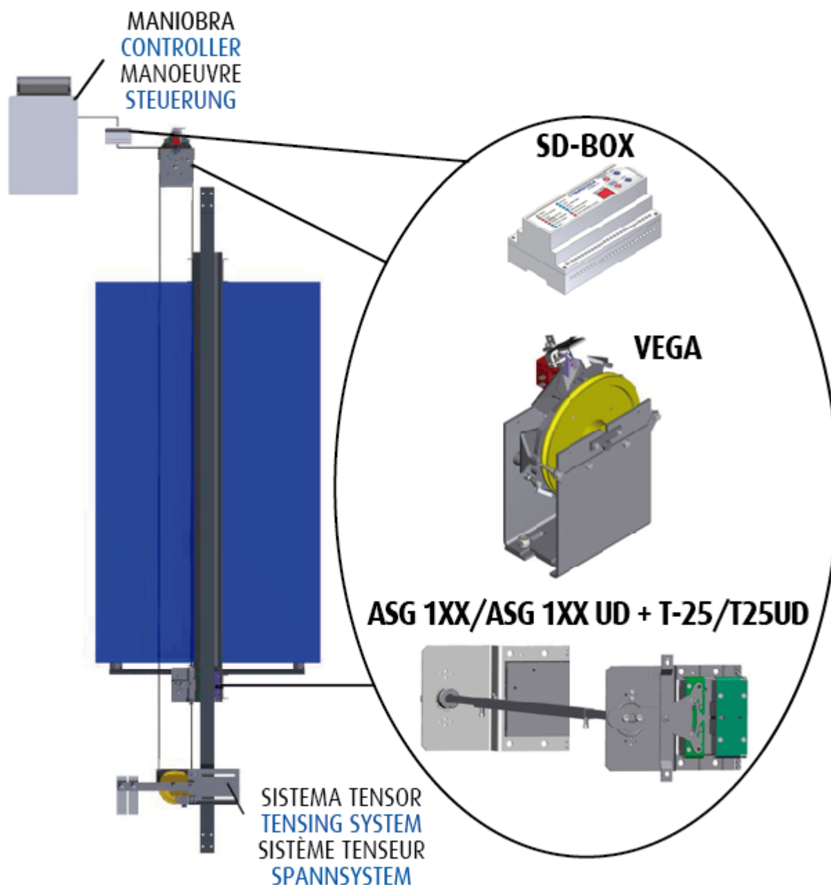
ABBILDUNG 2: Systemkomponenten
