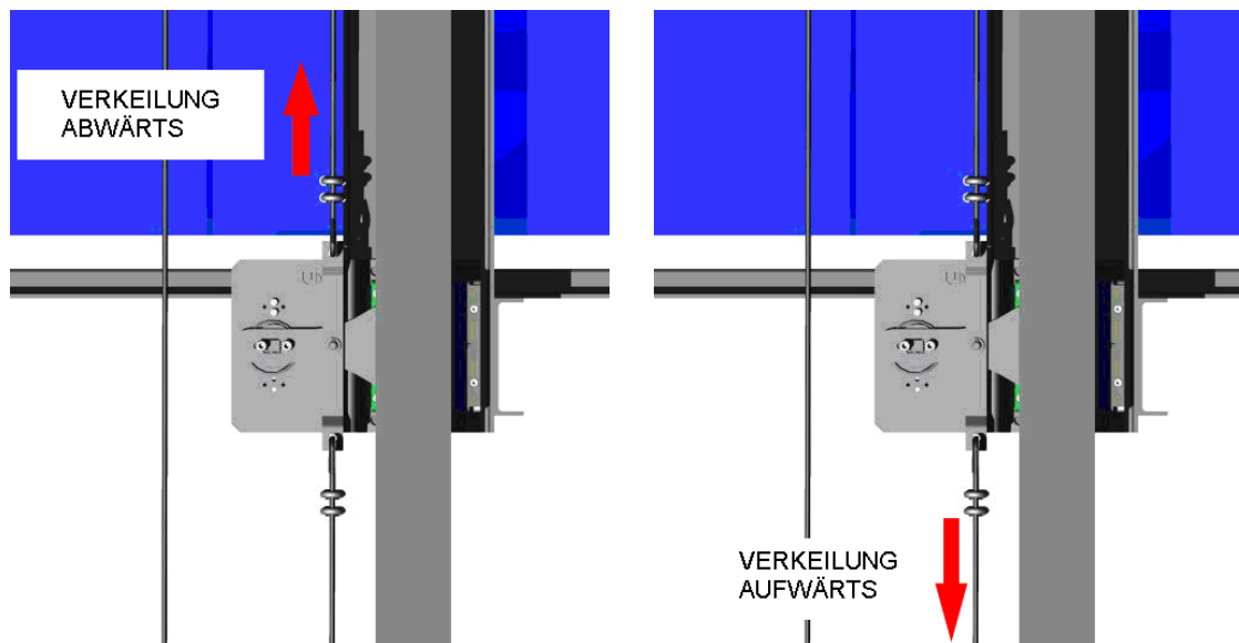
ABBILDUNG 5: Betätigung ASG 1XX + Auslösegestänge T-25
